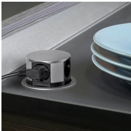
Emuca Multiconnettore Vertikal Push diametro 100mm, 3 spine di tipo Schuko, 1 USB tipo A, 1 USB tipo C, Acciaio e Tecno
