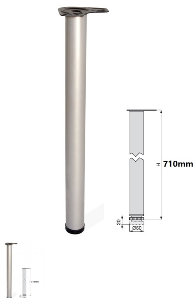
Gamba per Tavolo Silver Opaco diametro 60 mm regolabile
